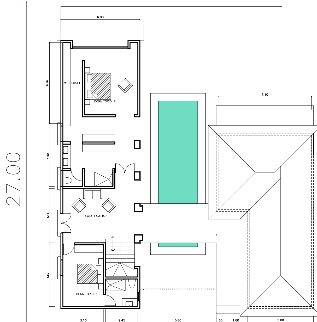
PLANTA AMUEBLADA 2DO NIVEL
