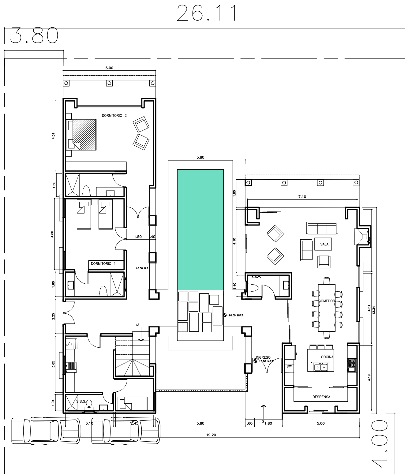
PLANTA AMUEBLADA 1ER NIVEL
